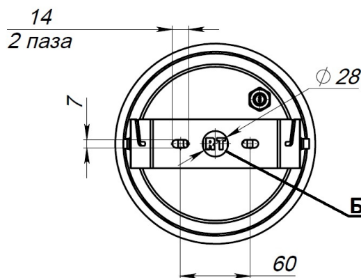
Установочные размеры
